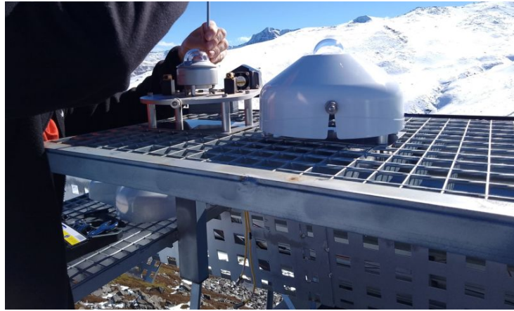
Radiómetros
