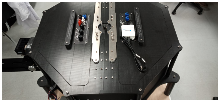
Nefelometro Polar
